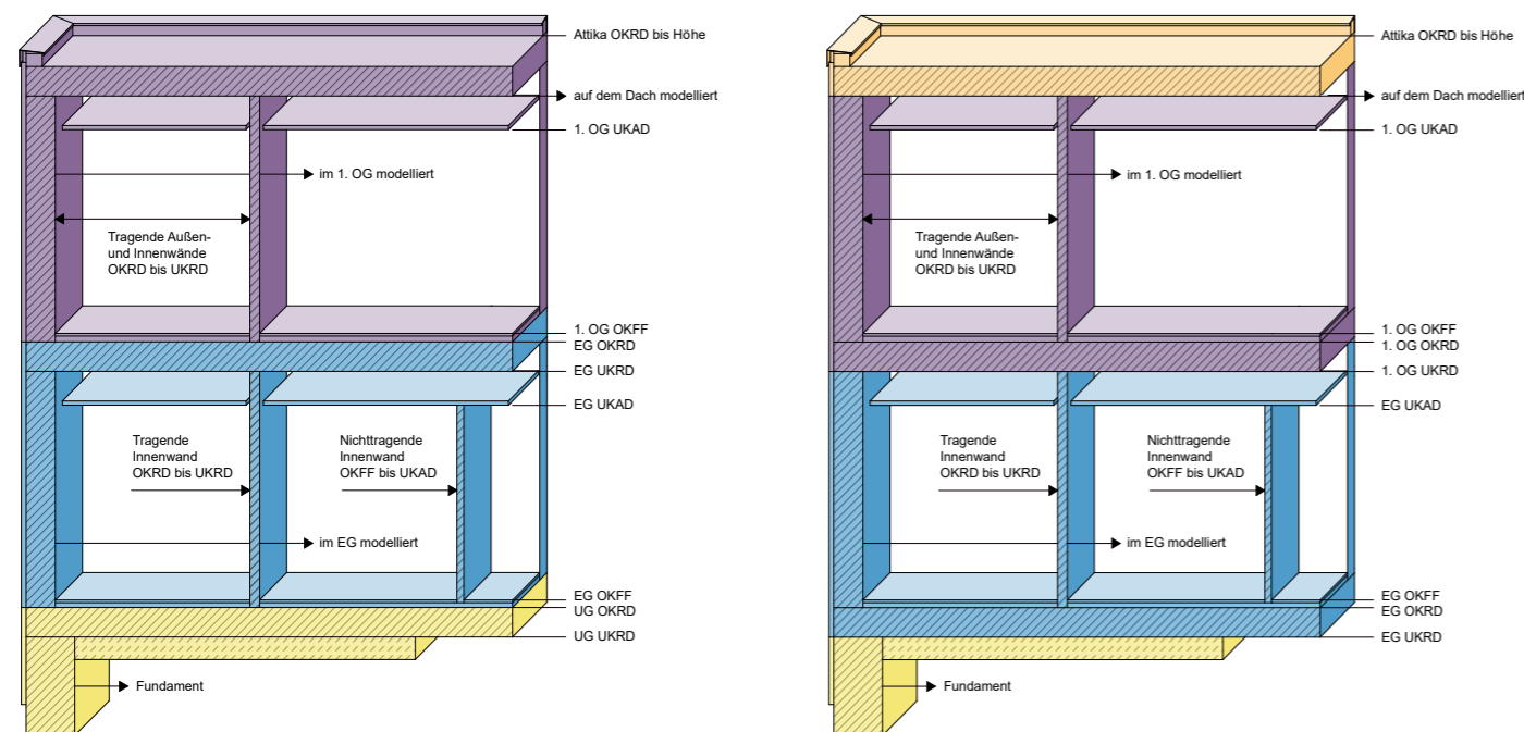
Abbildung 3: Geschossgliederung
